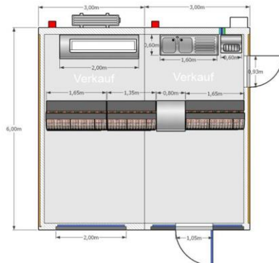
2er Verkaufsanlage 6x6m
