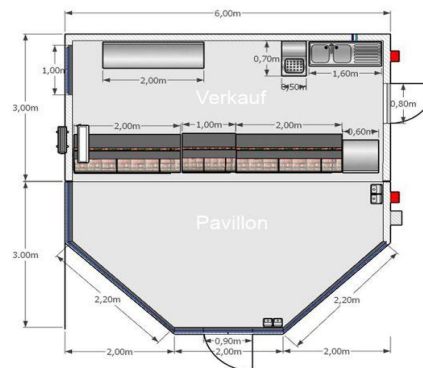
2er Verkaufsanlage 6x6m
