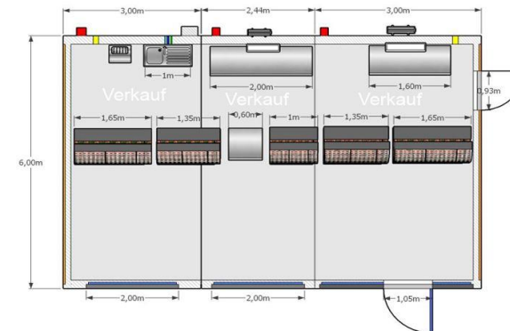
3er Verkaufsanlage 9x6m
