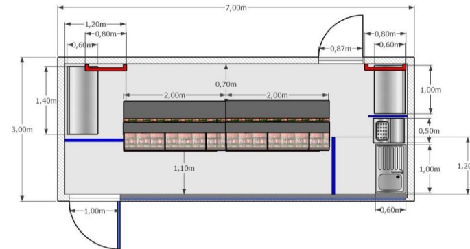
Verkaufsmodul 7x3m
