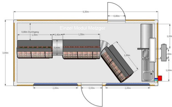
Verkaufsmodul 6,5x3m
