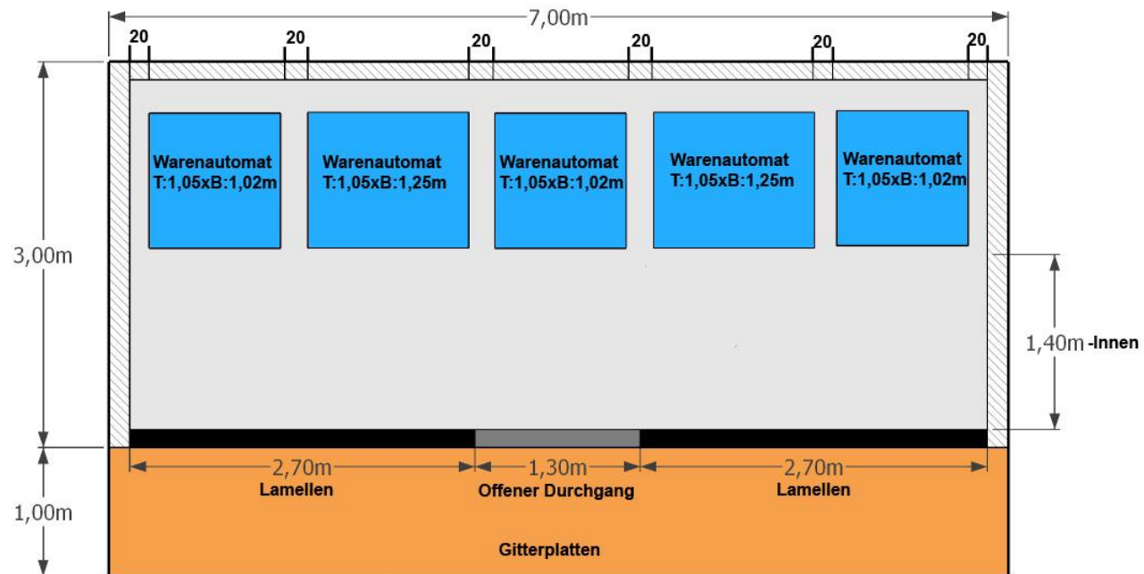
24/7 Verkaufsmodul 7x3m
